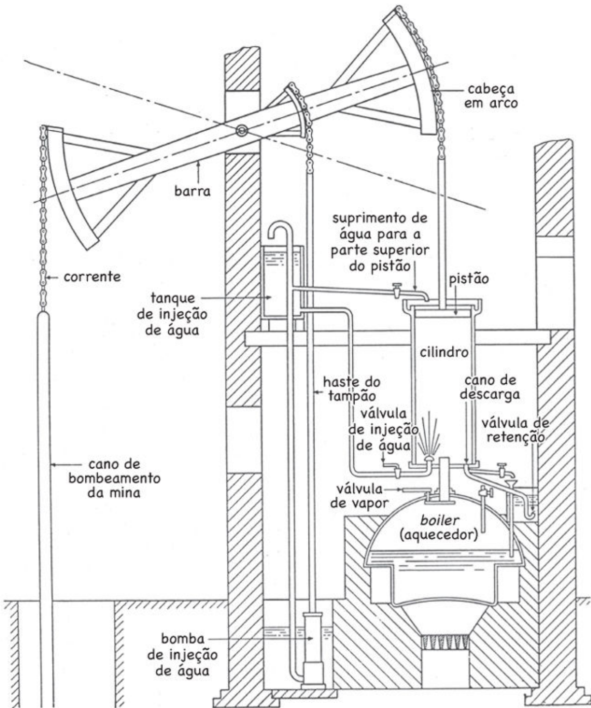
FIGURA 21: Motor a vapor atmosférico de Newcomen.
