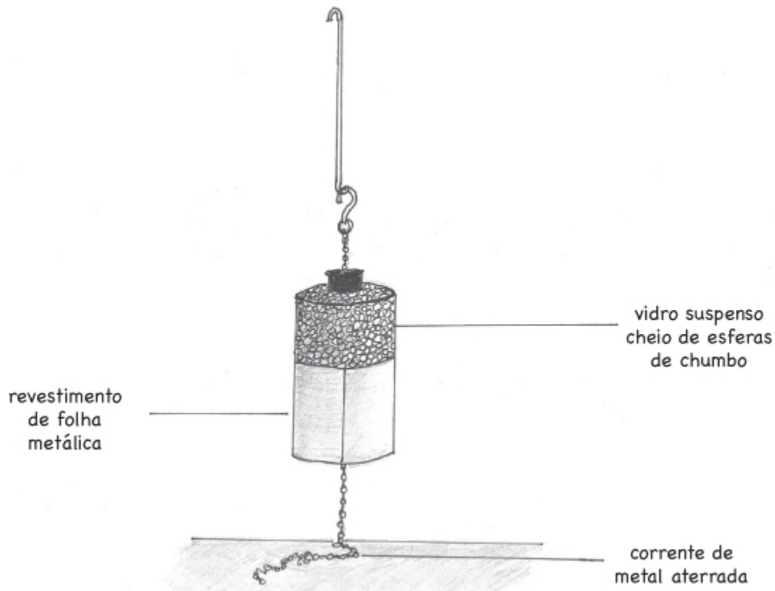
FIGURA 25: Garrafa de Leiden.
