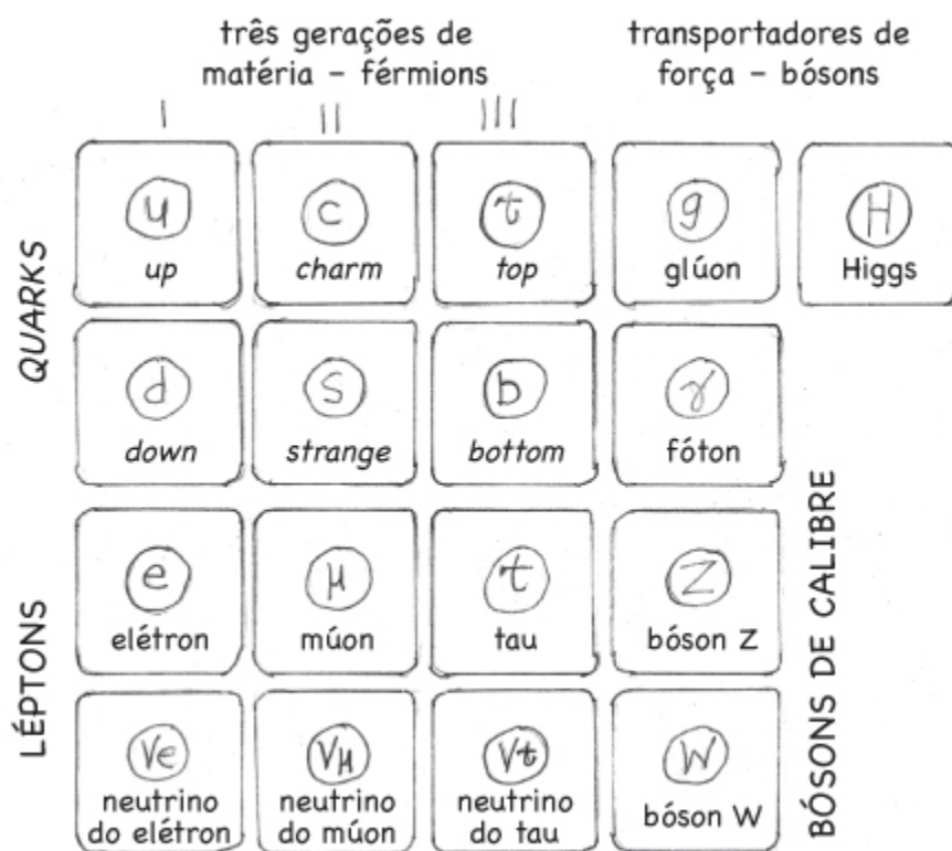
FIGURA 37: Modelo-padrão da física de partículas.
