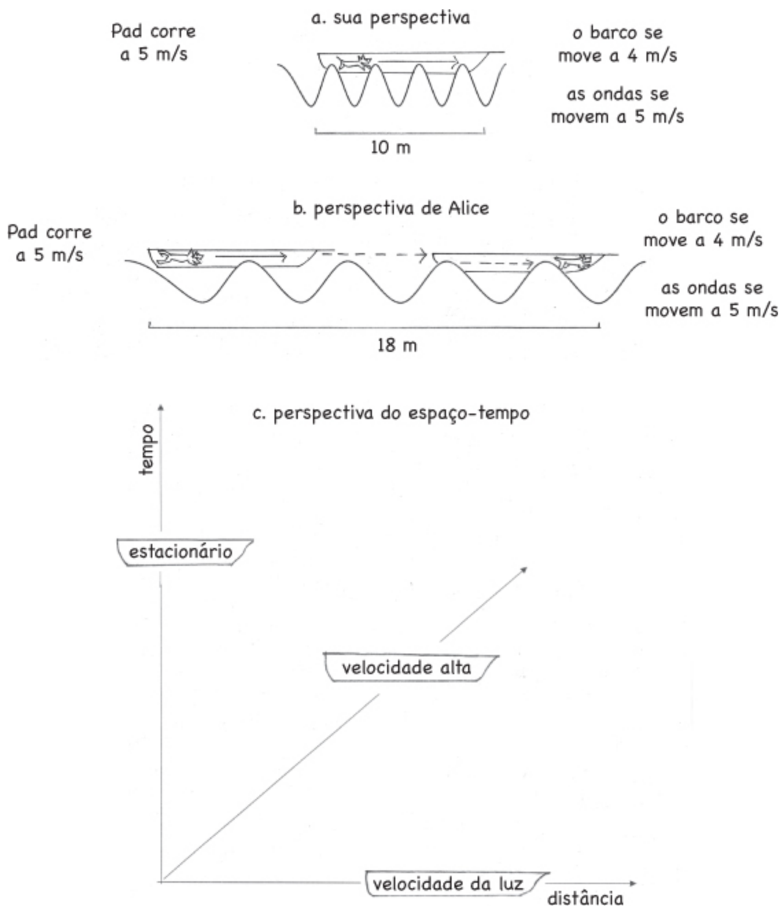
FIGURA 33: Relatividade especial em um barco.
