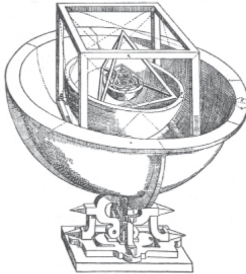
FIGURA 13: Modelo dos sólidos platônicos de Kepler para o sistema solar. O diagrama mostra um esquema do modelo do sistema solar ilustrando o aninhamento dos sólidos platônicos dentro das órbitas planetárias. Embaixo, há a ilustração de um modelo extraído do livro publicado por Kepler em 1596, Mysterium cosmographicum , que ele havia planejado construir com a forma de uma tigela de prata.
