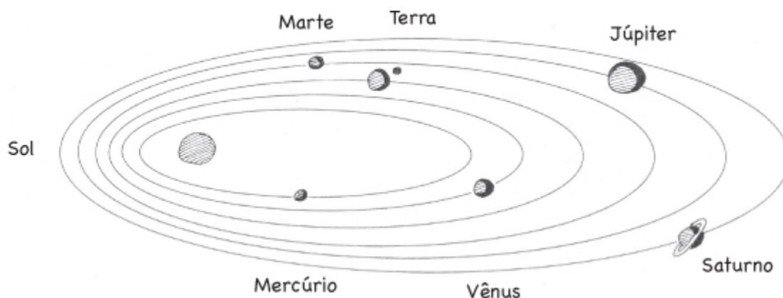
FIGURA 15: Sistema solar de Kepler com suas órbitas elípticas.
