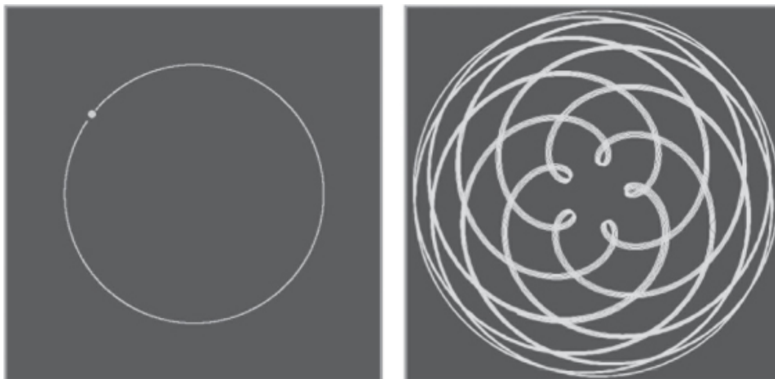
FIGURA 34: Perspectiva heliocêntrica (esquerda) versus geocêntrica (direita) da órbita de Vênus ao longo de um período de 32 anos. Com o Sol no centro, a órbita de Vênus é o círculo perfeito na figura à esquerda.
