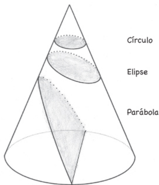
FIGURA 14: Seções cônicas.
