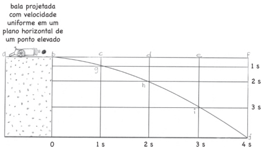
FIGURA 17: Análise do movimento de um projétil feita por Galileu.
