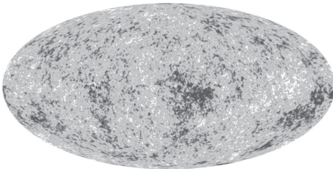
FIGURA 2: Radiação cósmica de fundo em micro-ondas.
