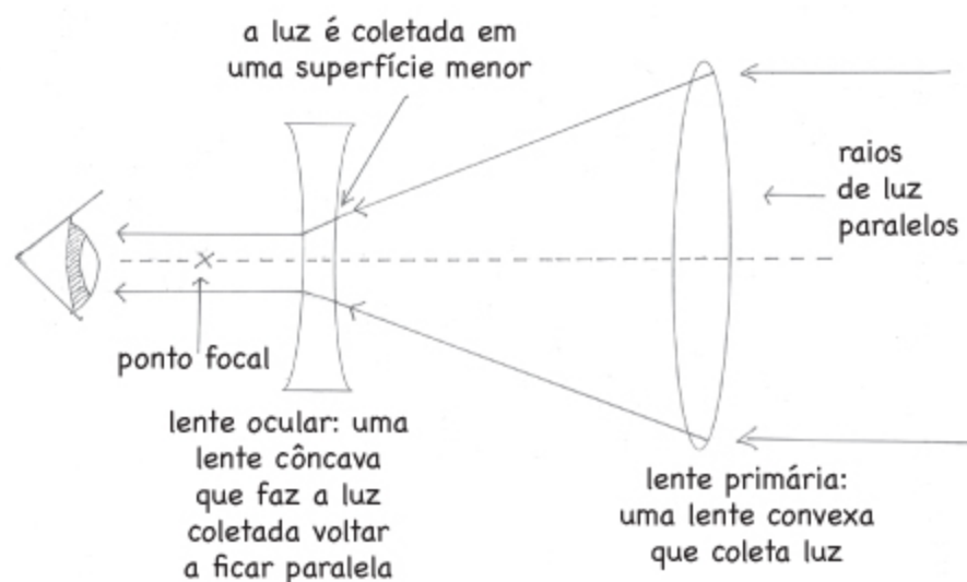
FIGURA 16: Princípio do telescópio refrator.
