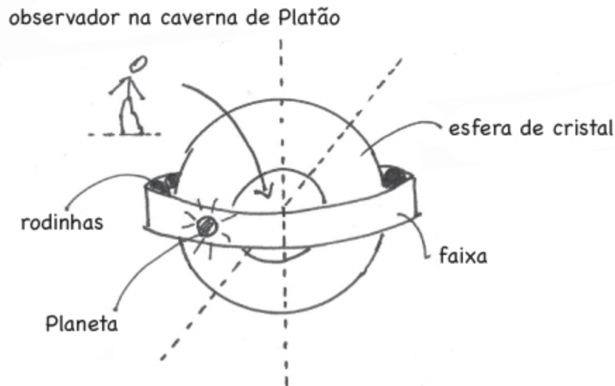
FIGURA 5: Vista dos movimentos planetários no modelo de Eudoxo.
