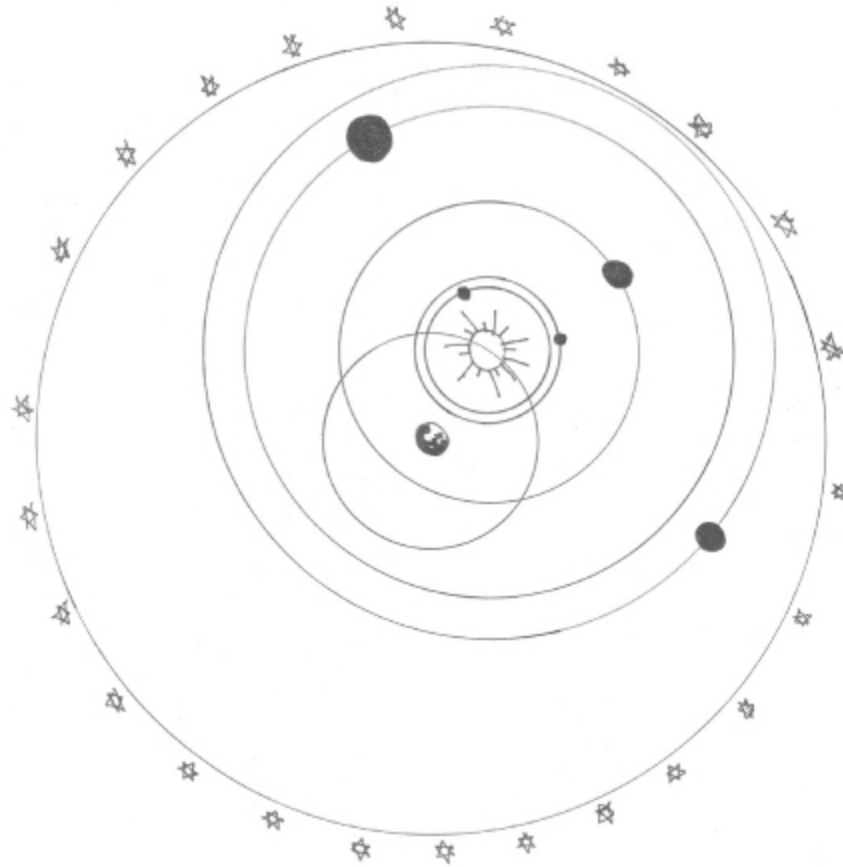
FIGURA 12: Sistema geo-heliocêntrico de Brahe.
