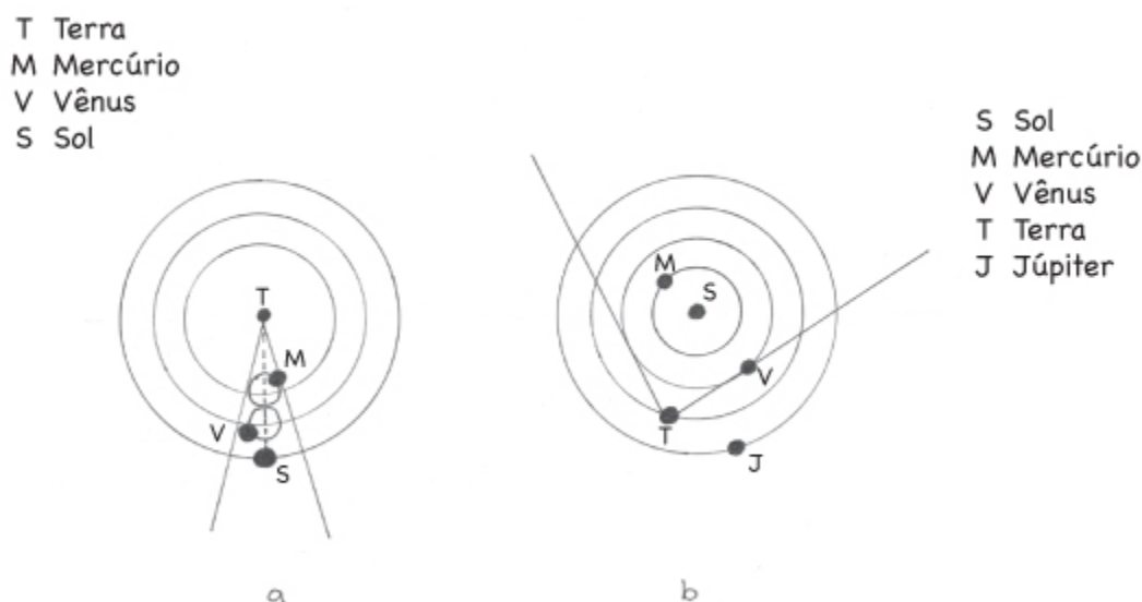
FIGURA 9: Perspectiva dos planetas a partir da Terra em um sistema (a) geocêntrico ou (b) heliocêntrico.
