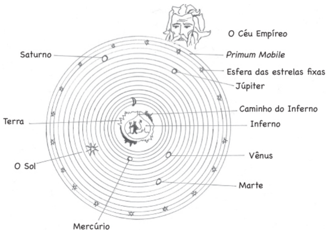
FIGURA 3: O cosmo medieval.
