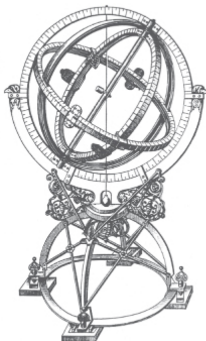
FIGURA 11: Esfera armilar.
