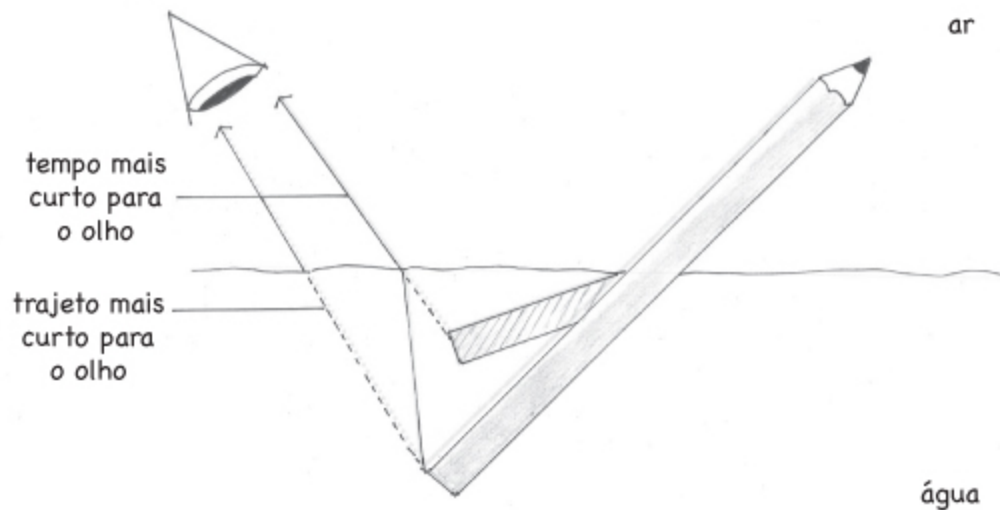
FIGURA 40: O princípio da mínima ação explica a aparente dobradura de um lápis parcialmente submerso.
