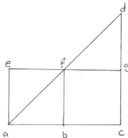
FIGURA 7: Prova gráfica do teorema de velocidade média feita por Buridan. O eixo horizontal ac é “tempo” e o eixo vertical cd é “velocidade acelerada” uniformemente, de modo que a distância total percorrida é dada pela área do triângulo adc . Buridan mostrou que, se o ponto f for equidistante de a e d , o triângulo fdg tem o mesmo tamanho do triângulo aef , uma vez que o retângulo aegc tem a mesma área do triângulo adc . Mas essa área é igual à distância percorrida viajando a uma velocidade média.
