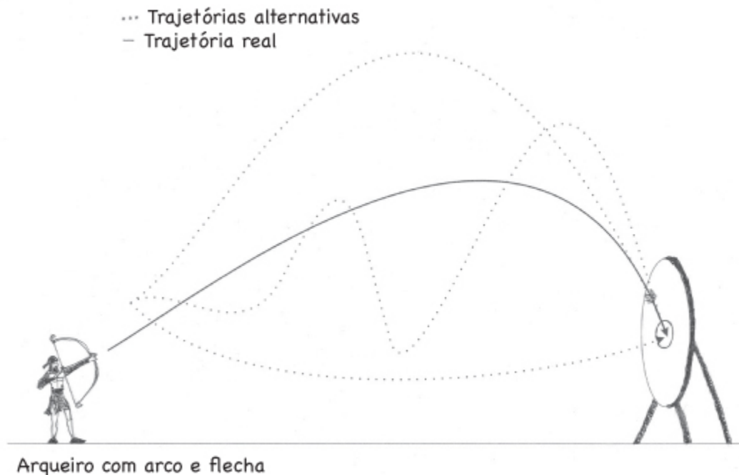
FIGURA 41: O princípio da mínima ação explica a trajetória parabólica de projéteis como flechas.
